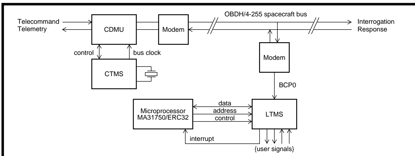
Figure A.3 - OB DH 4-255 Data Bus Application
