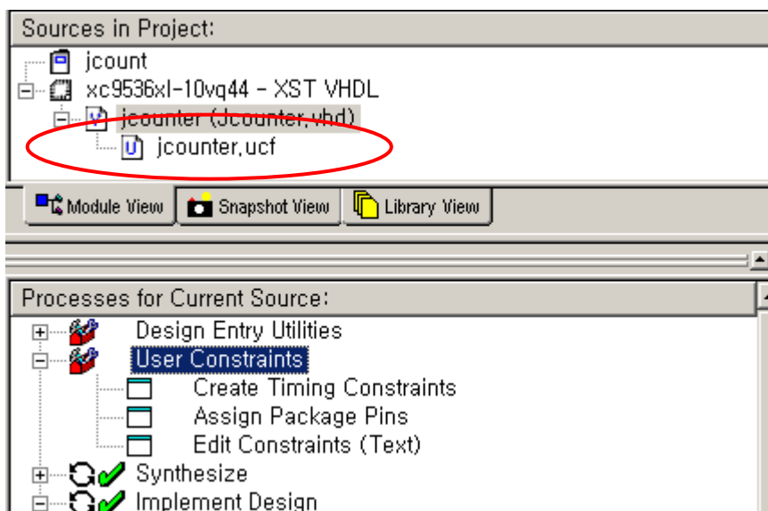
< 그림 23 > User Constraints
